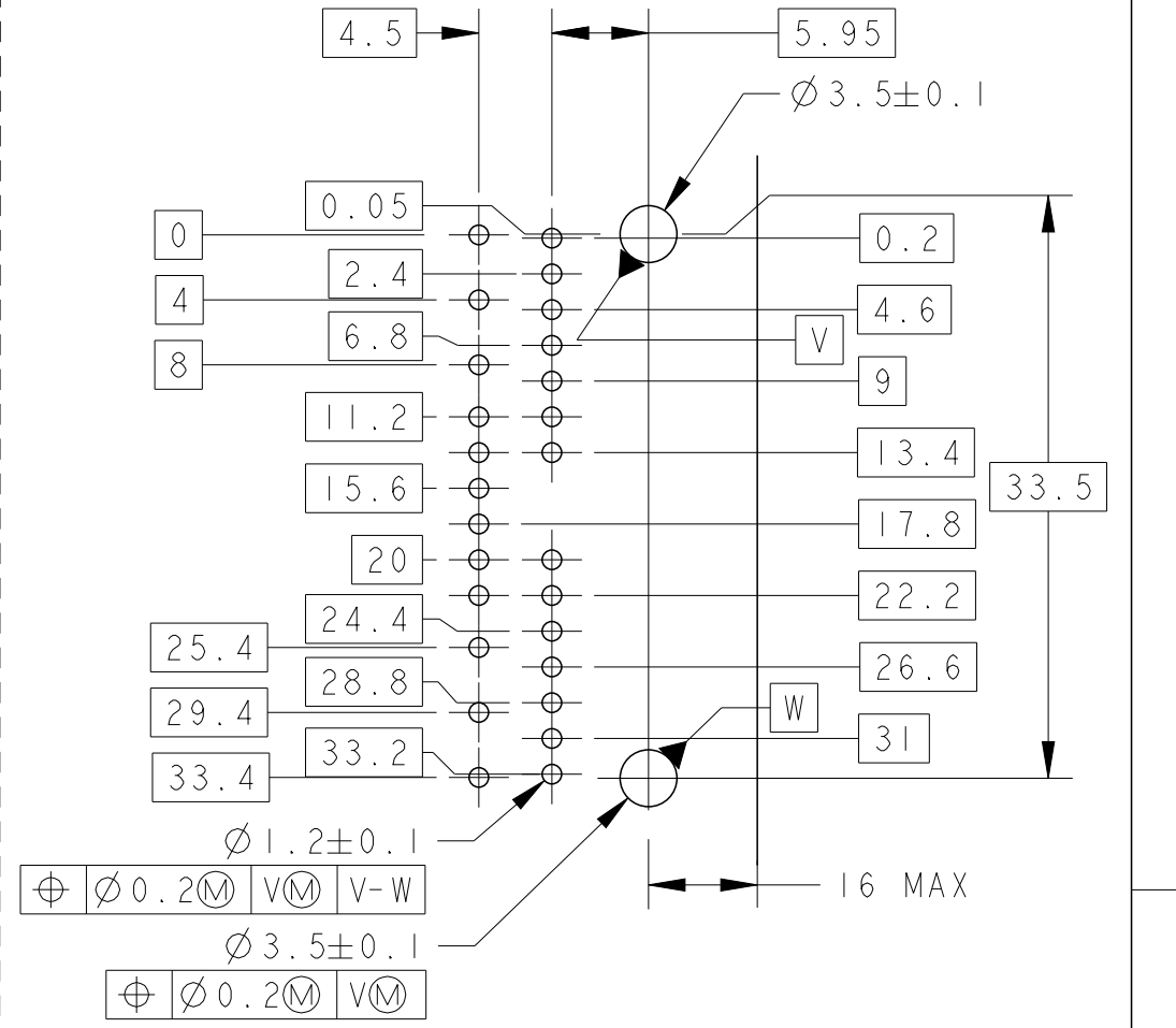
プリント基板取付寸法図 DIMENSION FOR P.C. BOARD
