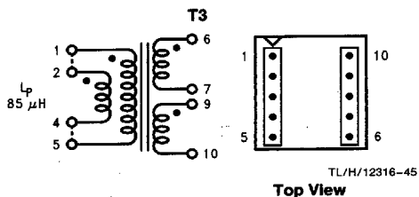
FIGURE 31. Schott 67140920
