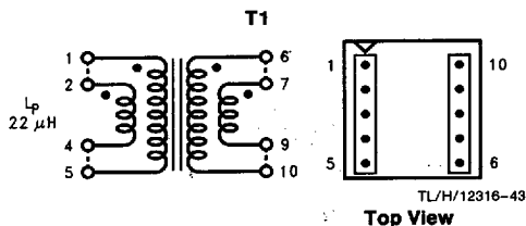
FIGURE 29. Schott 67141450
