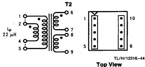
FIGURE 30. Schott 67140860
