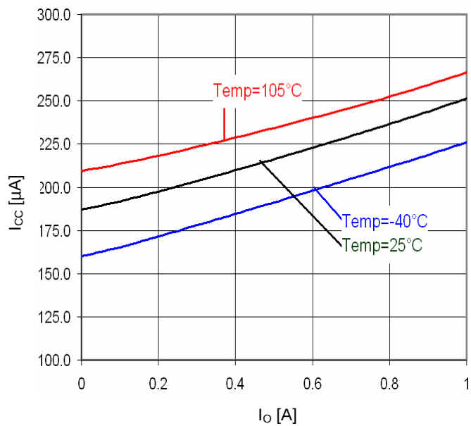
Fig.32 Io-Icc
