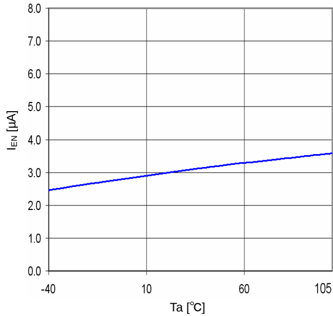
Fig.24 T_a - I_{EN}
