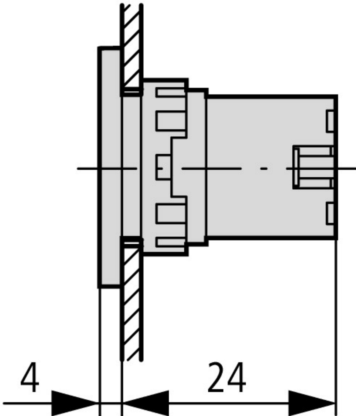
Betätigungs- und Signalisierungselemente Quadratisches Design
