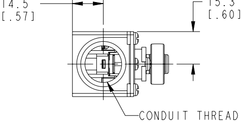
Figure 22. GLD Conduit
