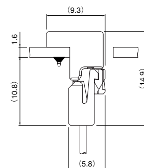
PAF Receptacle + PA bottom type header
