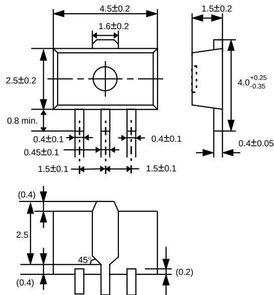
(3) SOT-89-3
