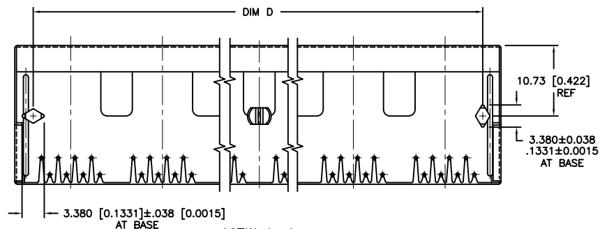
VIEW A-A
