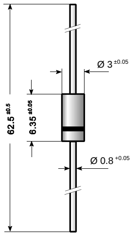
Dimensions / Maße in mm
