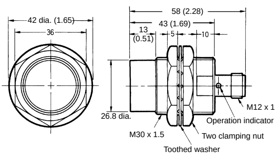
Fig. 19: E2E-X18ME□-M1/F□-M1-N
