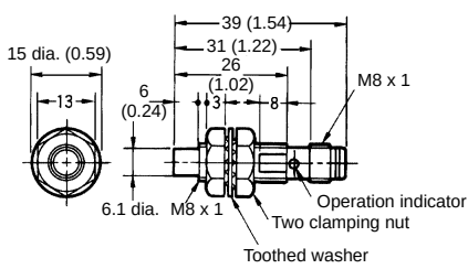
Fig. 21: E2E-X2ME□-M3/F□-M3-N
