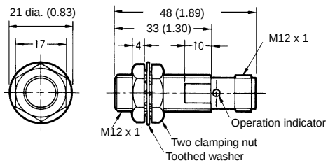
Fig. 16: E2E-X5E□-M1/F□-M1-N
