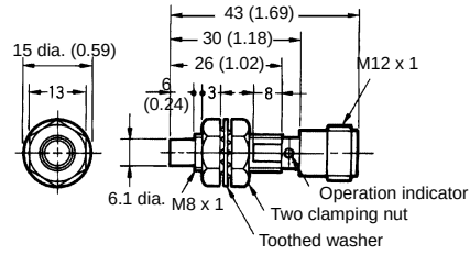
Fig. 13: E2E-X2ME□-M1/F□-M1-N
