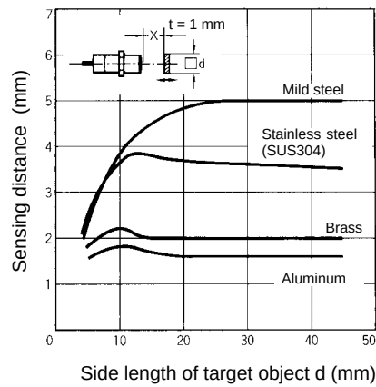
E2E-X5ME□/F□-N
