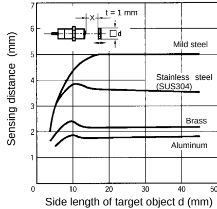
E2E-X5ME□/F□-N
