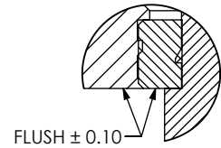
DETAIL 'B' SCALE 15:1
