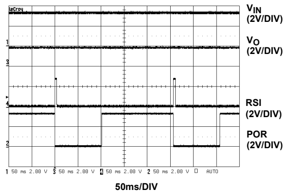
FIGURE 7. POR FUNCTION
