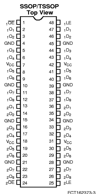
FCT162373-3
