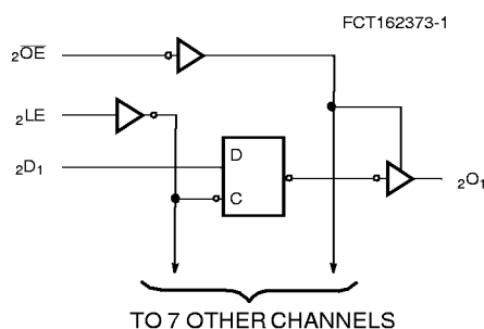
FCT162373-2
