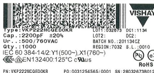
PN: VKP222MCQEDOKR
