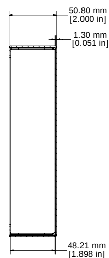
SECTION A-A
