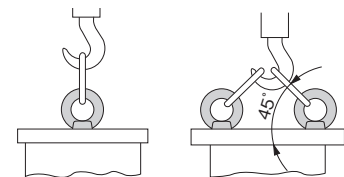
垂直つり Vertical suspending 45度つり 45° suspending
