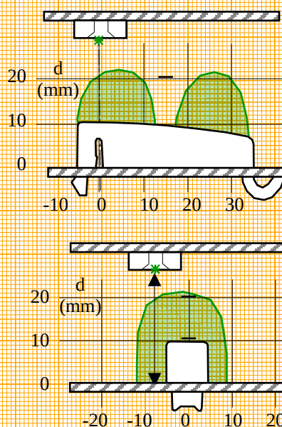
Vis/Screw M4 max
