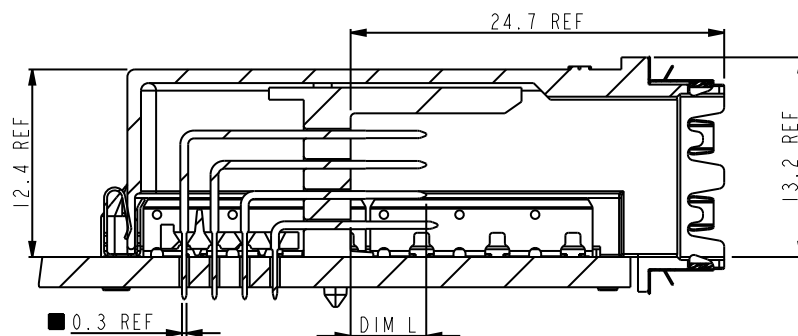
SECTION A-A SCALE 2.000
