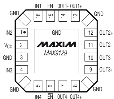
QFN
