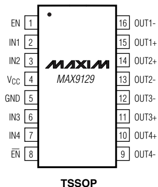
TSSOP
