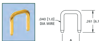
.040 (1.0) PINS
