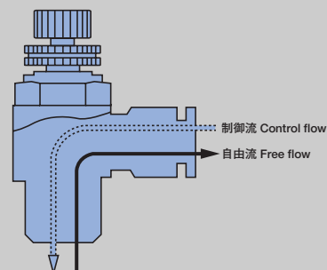
メーターイン制御 Meter-in control
