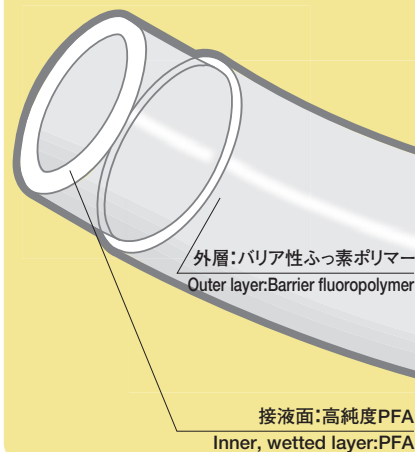
チューブ構造図/Structure
