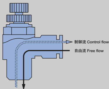
メーターアウト制御 Meter-out control
