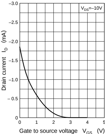
I_D - V_{GS}
