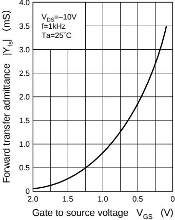
|Y_{fs}| - V_{GS}
