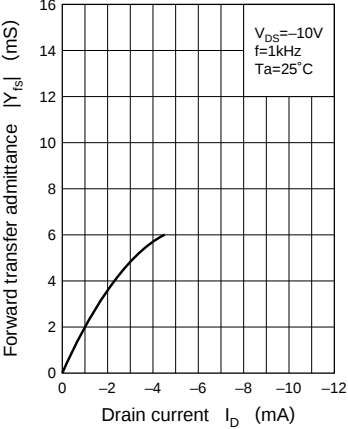
|Y_{fs}| - I_D
