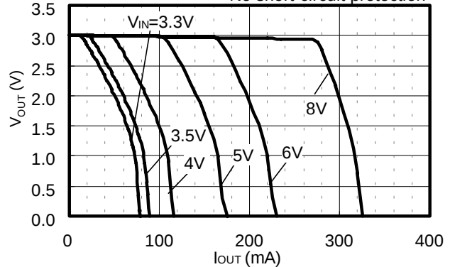
S-812C30A (Ta=25°C)
