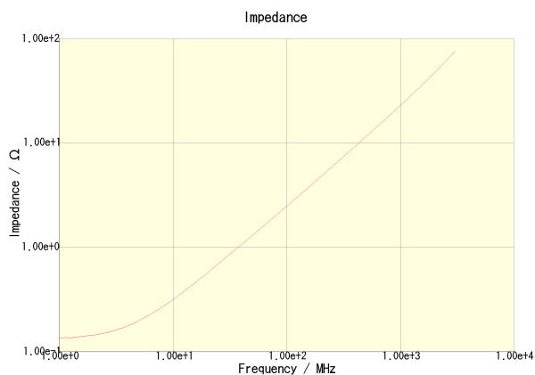
MLK1005S3N9ST000
