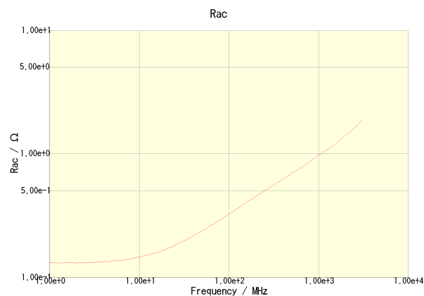
MLK1005S3N9ST000
