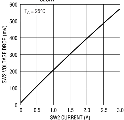
SW2 V_{\text{CESAT}}
