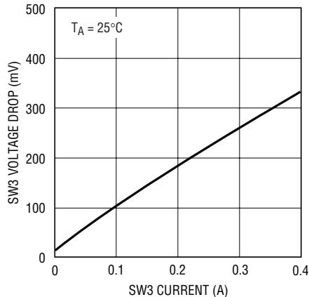
SW3 V_{\text{CESAT}}
