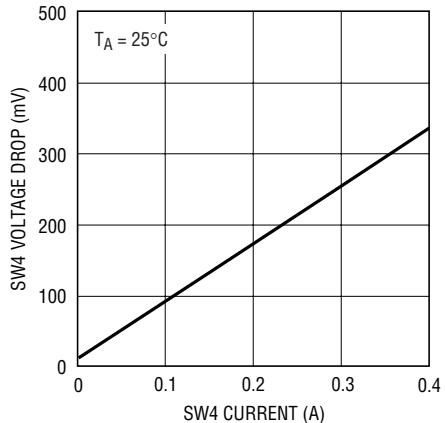
SW4 V_{\text{CESAT}}
