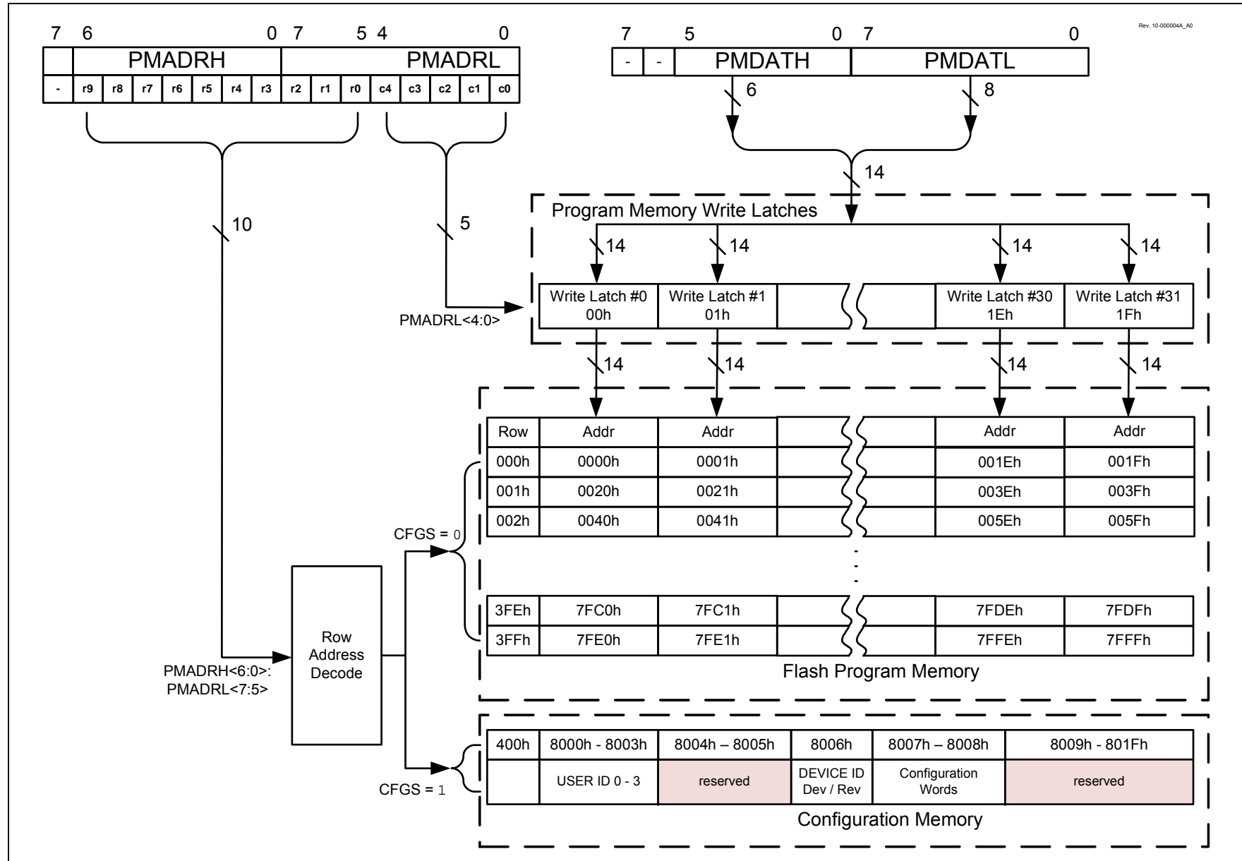
PIC16(L)F1704/8
