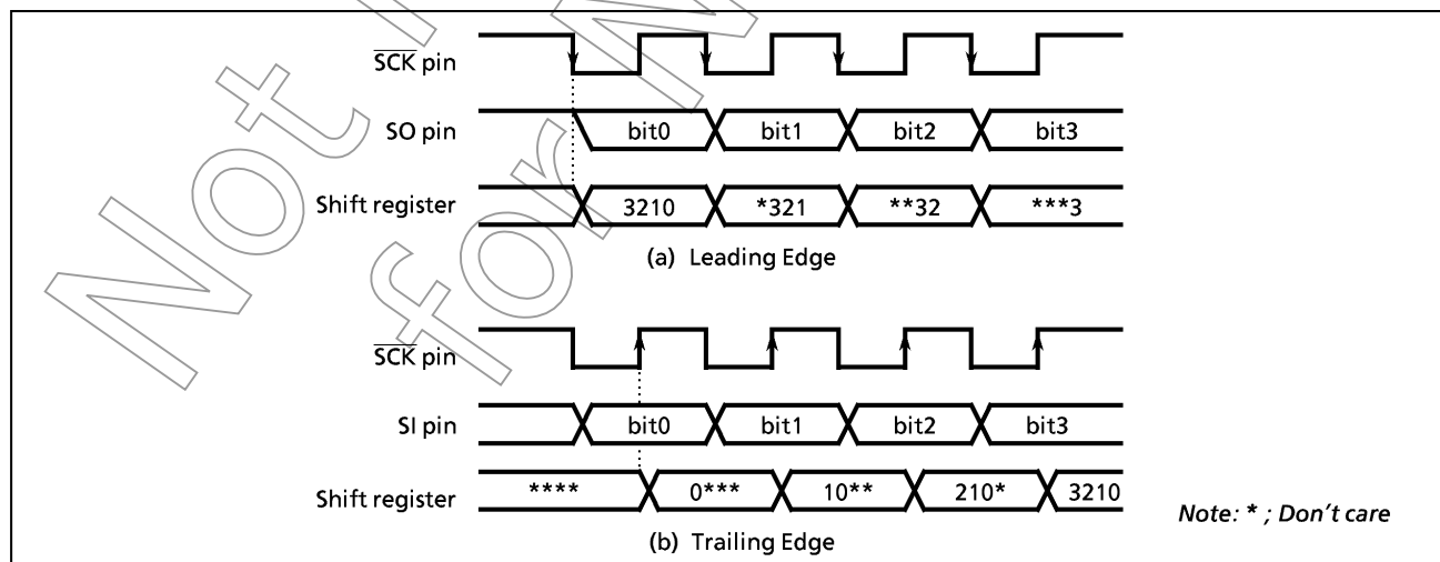
Figure 2-36. Shift Edge
