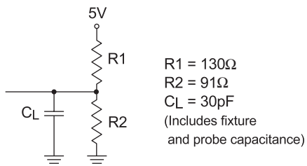
TTL AC Test Load (16)
