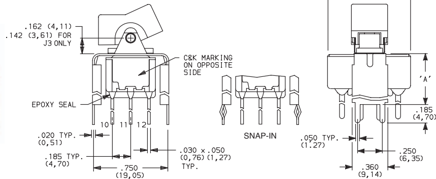
7401J1_BE2 4PDT
