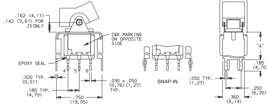
7201J1_BE2 DPDT
