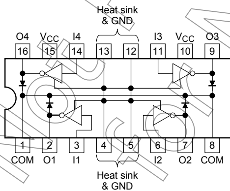
TD62164APG
