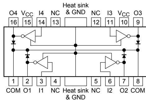
TD62164AFG
