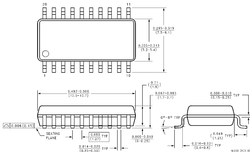
20-Lead Plastic EIAJ SOIC (SJ) Package Number M20D
