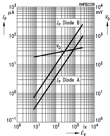
Photocurrent / Open-Circuit Voltage Fotostrom / Leerlaufspannung I_P (V_R = 5 \text{ V}) / V_O = f(E_V)
