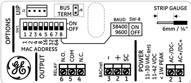
BACnet Wiring
