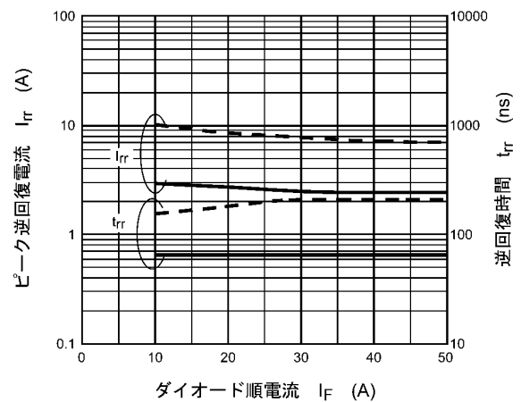
図 8.18 I_R , t_{rr} - I_F
