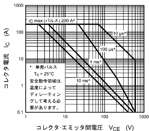
図 8.19 安全動作領域 (最大値 (保証値))
