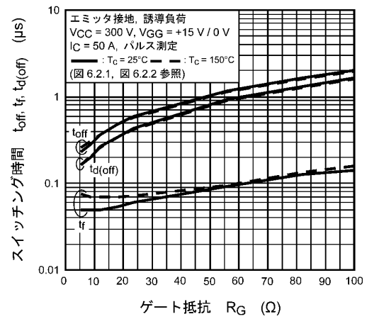
図 8.12 t_{off}, t_r, t_d(off) - R_G
