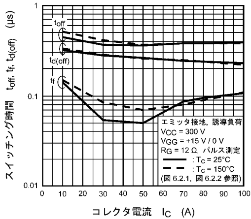
図 8.13 t_{off} , t_r , t_d(off) - I_C
