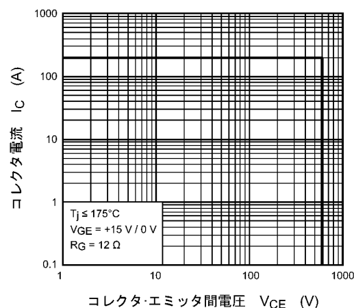
図 8.20 逆バイアス安全動作領域 (最大値 (保証値))
