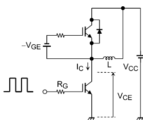
図 6.2.1 スwitchング時間の測定回路
