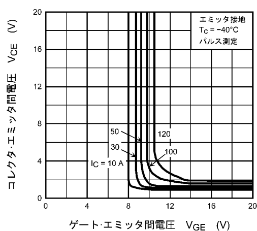
図 8.6 V_{CE} - V_{GE}
