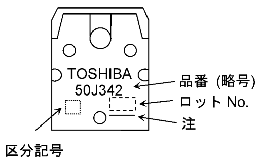
図 7.1 現品表示
