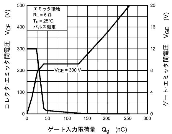
図 8.16 V_{CE} , V_{GE} - Q_g
