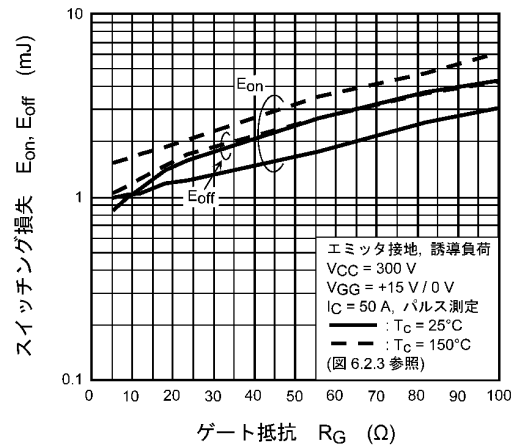
図 8.14 E_{on} , E_{off} - R_G
