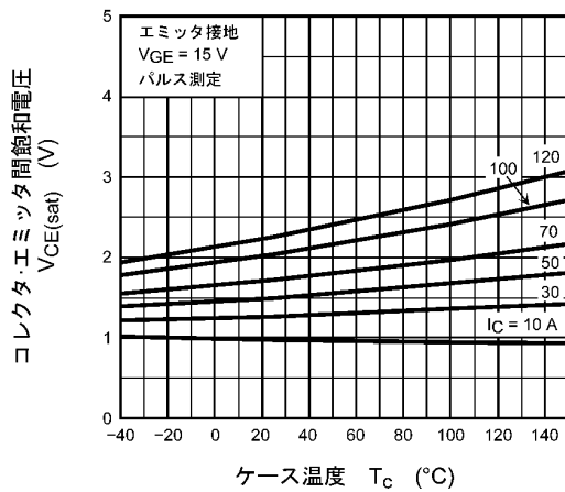
図 8.9 V_{CE(sat)} - T_c
