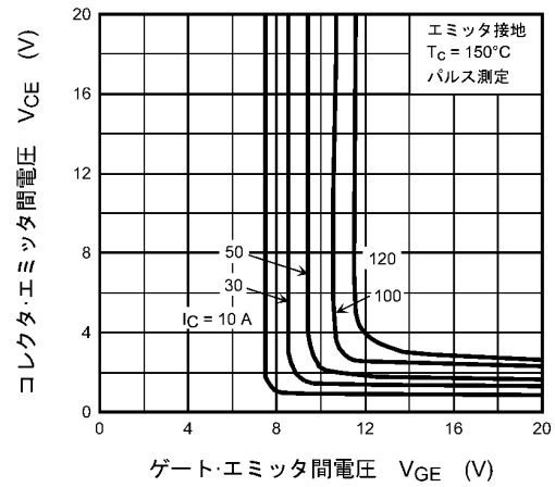
図 8.8 V_{CE} - V_{GE}
