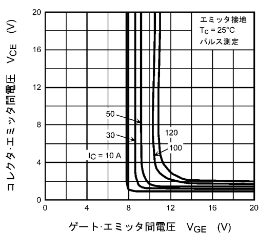
図 8.5 V_{CE} - V_{GE}
