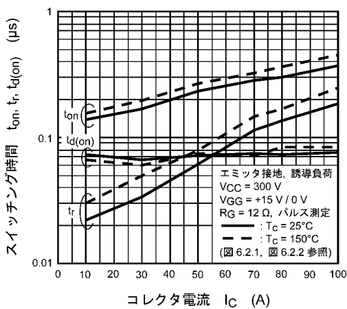
図 8.11 t_{on}, t_r, t_d(on) - I_C
