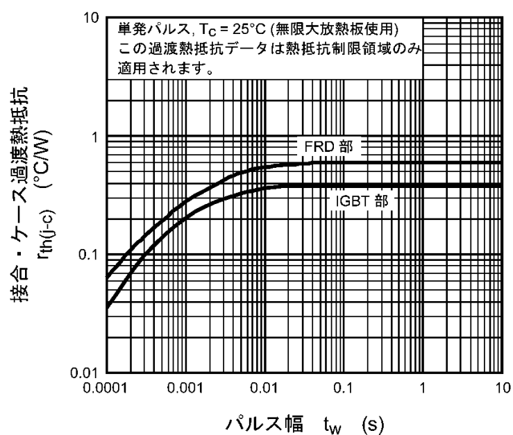
図 8.21 r_{th(j-c)} - t_w (最大値 (保証値))
