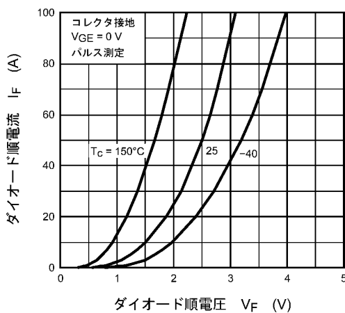
図 8.17 I_F - V_F
