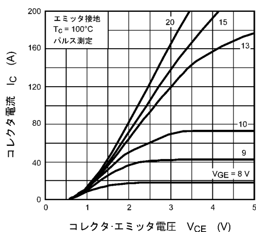
図 8.3 I_C - V_{CE}
