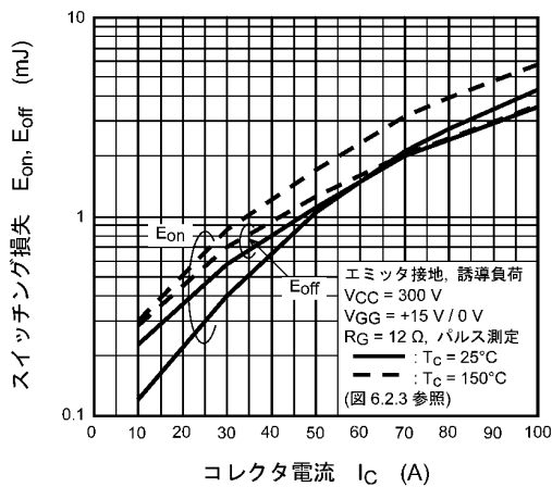
図 8.15 E_{on} , E_{off} - I_C
