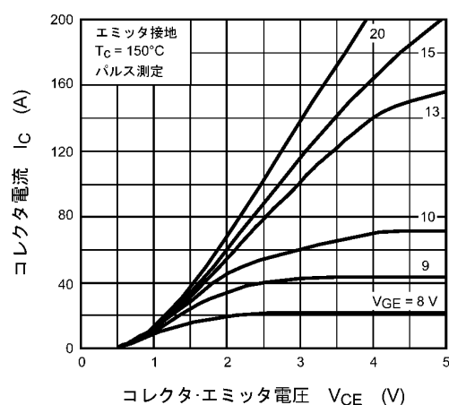
図 8.4 I_C - V_{CE}
