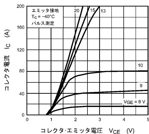
図 8.2 I_C - V_{CE}
