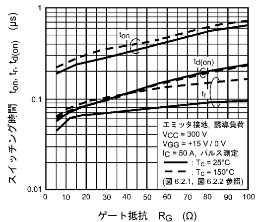
図 8.10 t_{on}, t_r, t_d(on) - R_G
