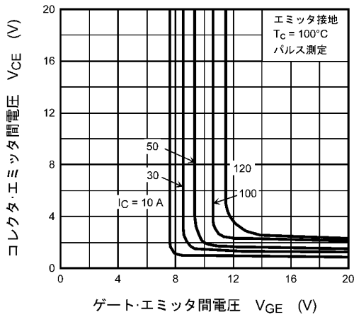
図 8.7 V_{CE} - V_{GE}
