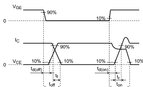
図 6.2.2 スwitchング時間のタイミングチャート
