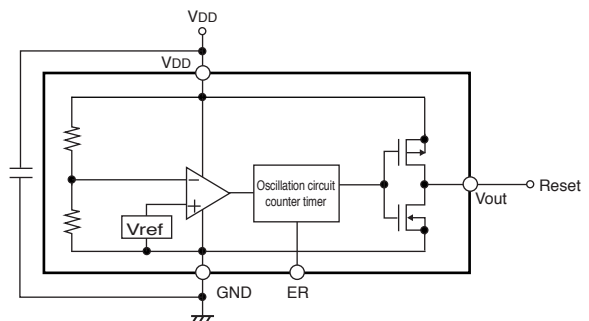
BD46XXXG
