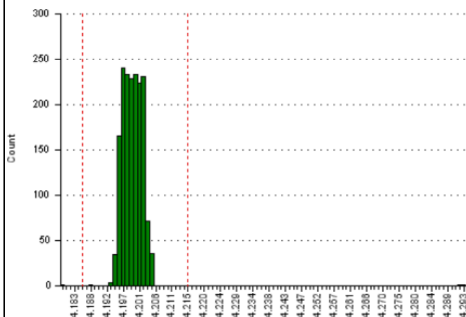
Const. Volt. Post trim
