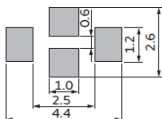
NFM31PC/31KC
