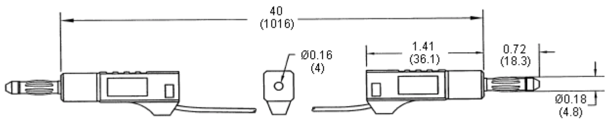
Dimensions : Inches (Millimetres)
