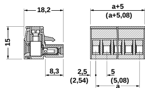
MSTB 2,5 HC/...-ST(-5,08)
