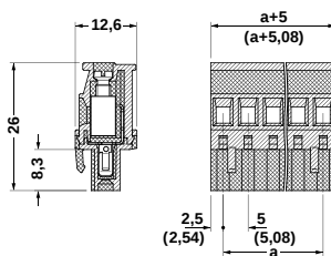
MVSTBR 2,5 HC/...-ST(-5,08)
