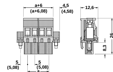
MVSTBW 2,5 HC/...-STF(-5,08)
