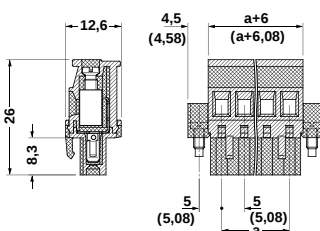
MVSTBR 2,5 HC/...-STF(-5,08)
