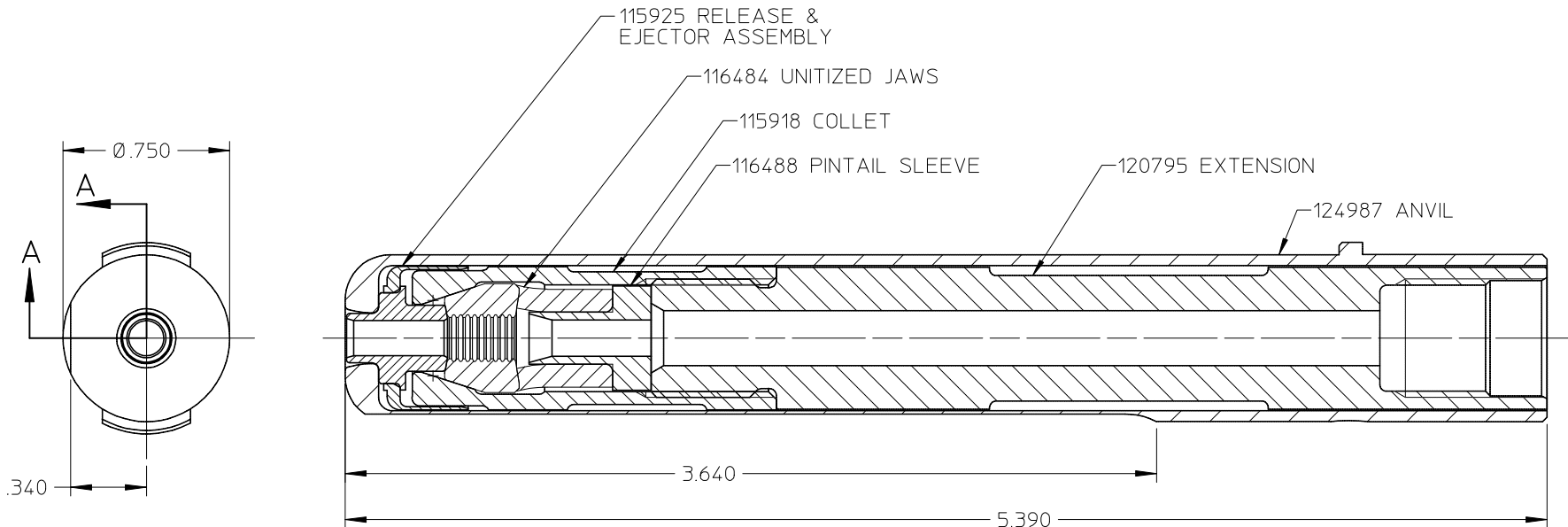
SECTION A-A
