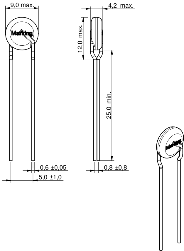
Scale - 2:1
