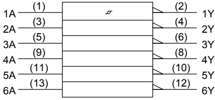
論理図
