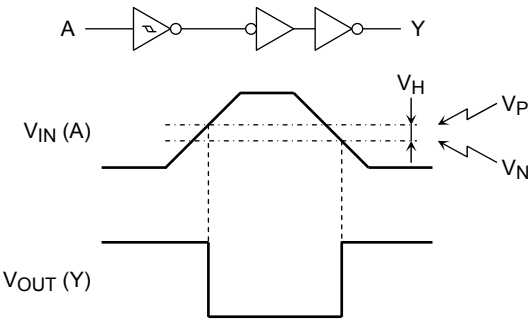
システム図・波形
