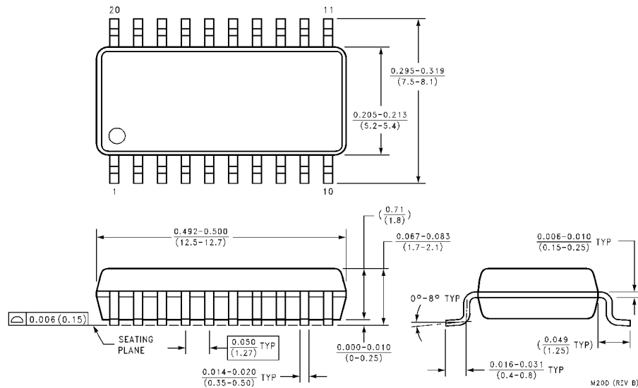
S.O. Package (SJ) Order Number DM74ALS244BSJ Package Number M20D
