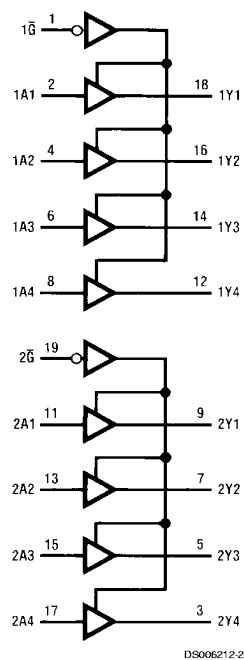
74ALS244A/74ALS244B
