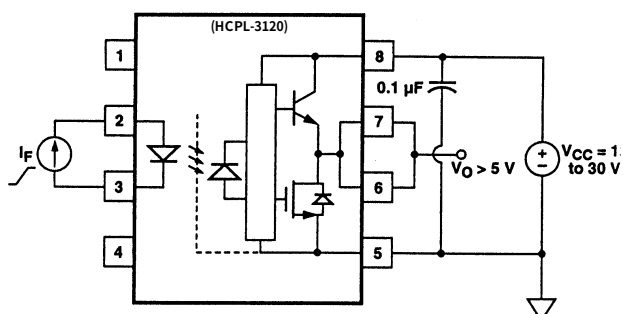
図21. I_{FILH} 試験回路
