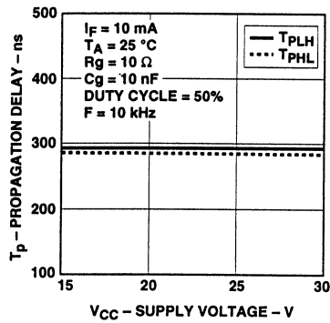
图10. 伝達遅延— V_{CC} 特性
