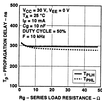
图13. 伝達遅延— R_g 特性
