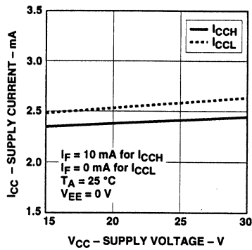
图8. I_{CC} — V_{CC} 特性
