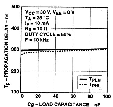
图14. 伝達遅延— C_g 特性
