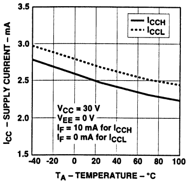
图7. I_{CC} —温度特性
