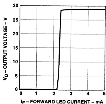
図15. I_F - V_O 伝達特性
