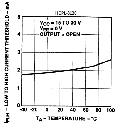
图9. I_{FLH} —温度特性
