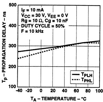
图12. 伝達遅延—温度特性
