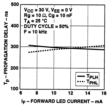
图11. 伝達遅延— I_F 特性
