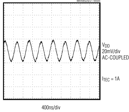
V_{DD} RIPPLE
