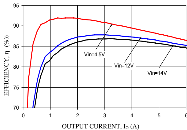
V_o = 1.8V
