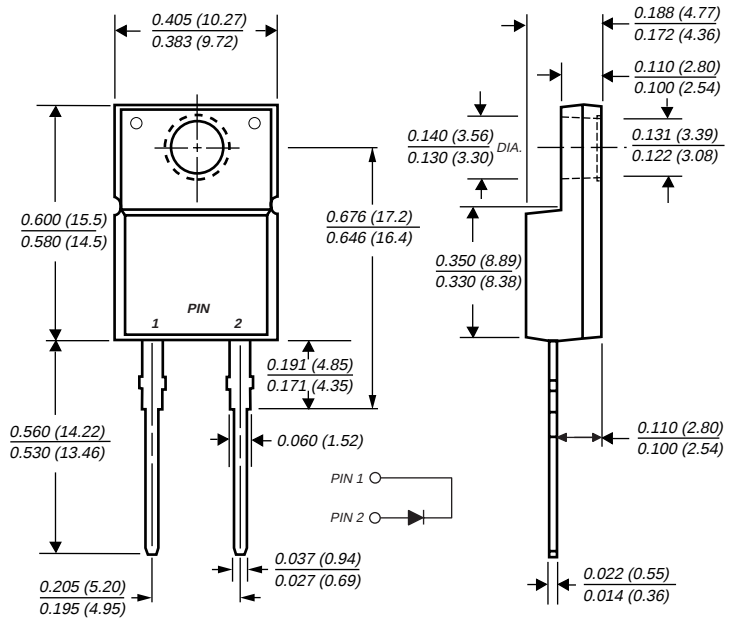
ITO-220AC (DTV32F)
