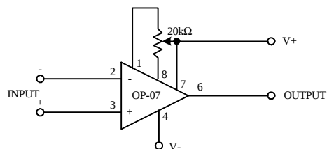
OPTIONAL OFFSET NULLING CIRCUIT
