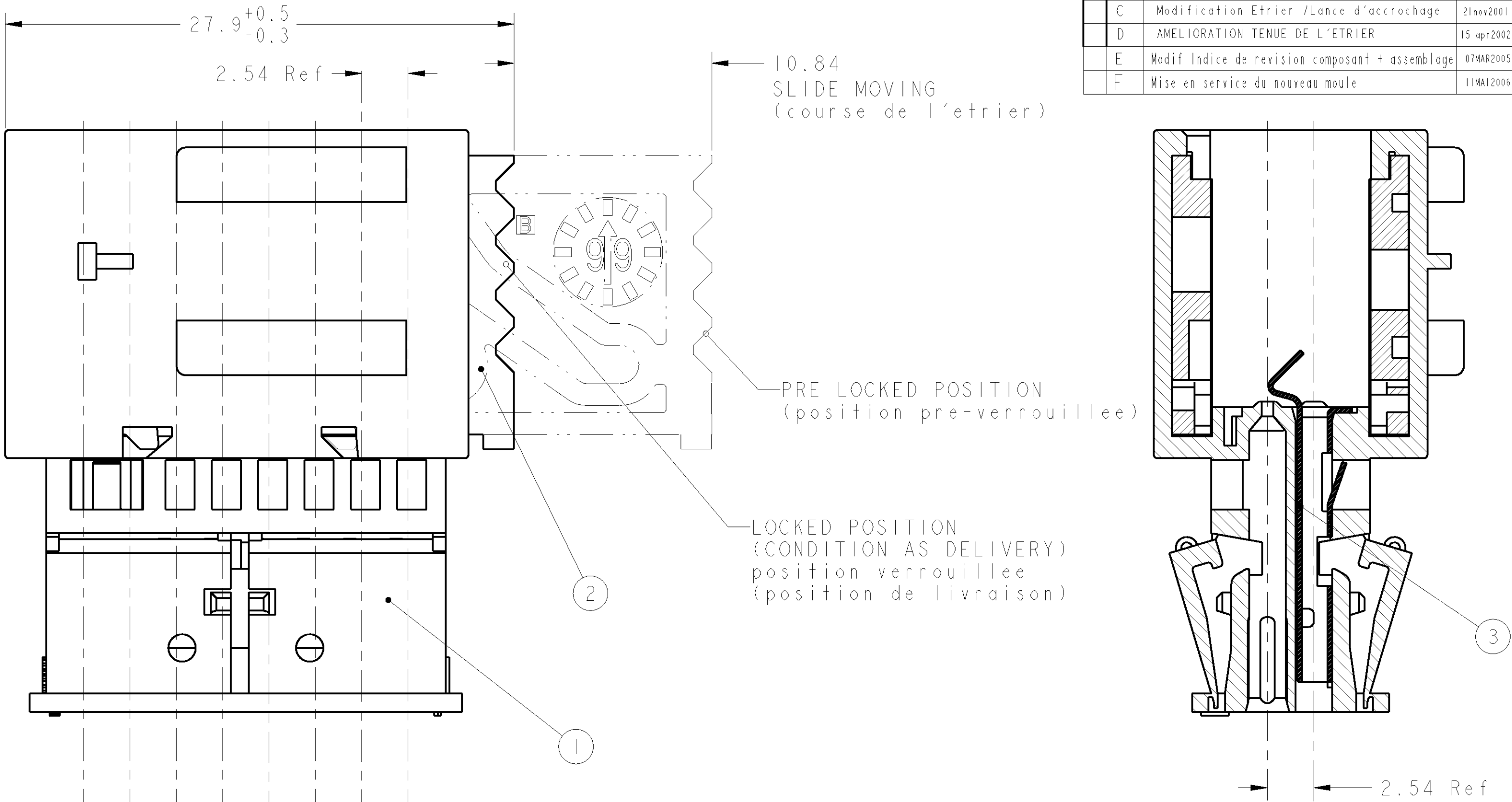
COUPE A-A EXCEPT FOR 953893-1 (excepte pour 953893-1)
