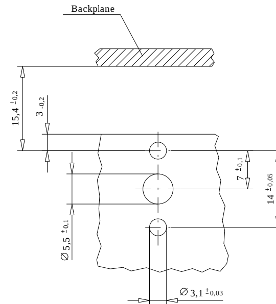
Layout der Tochterkarte - Layout of daughtercard
